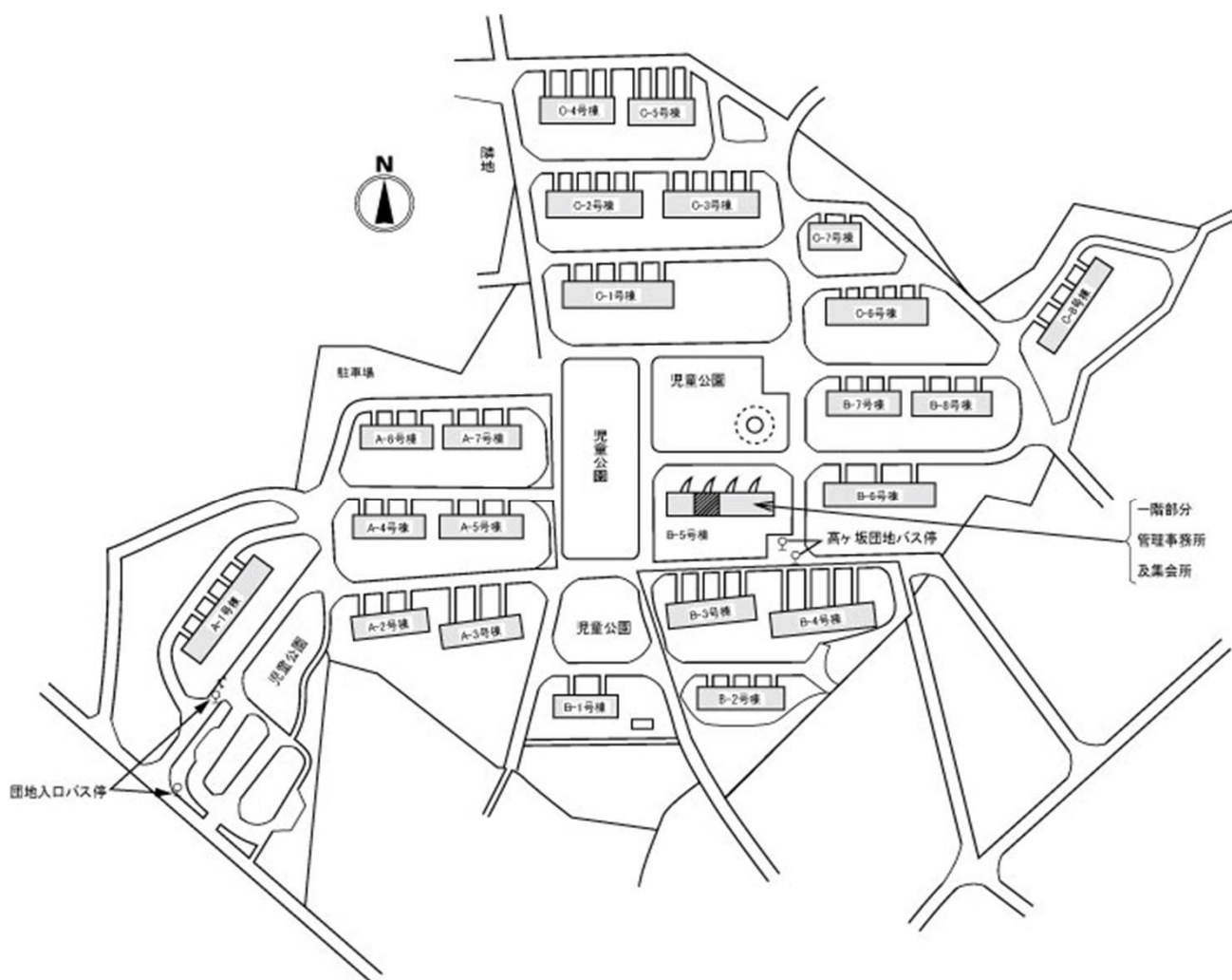
配置図
