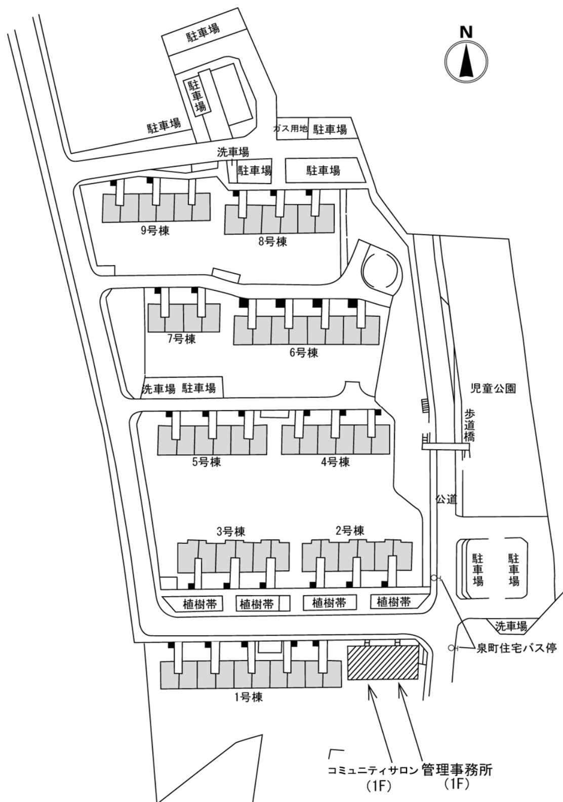
配置図
