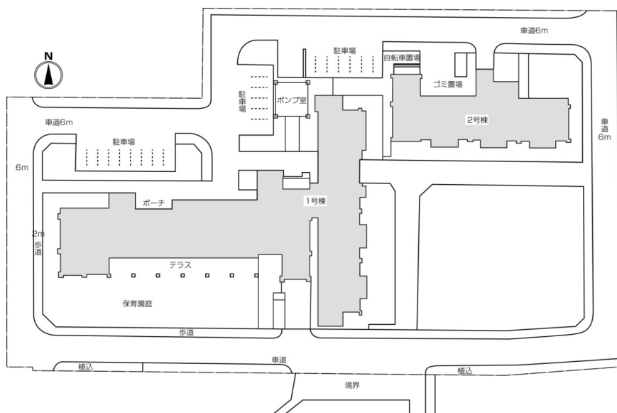
配置図
