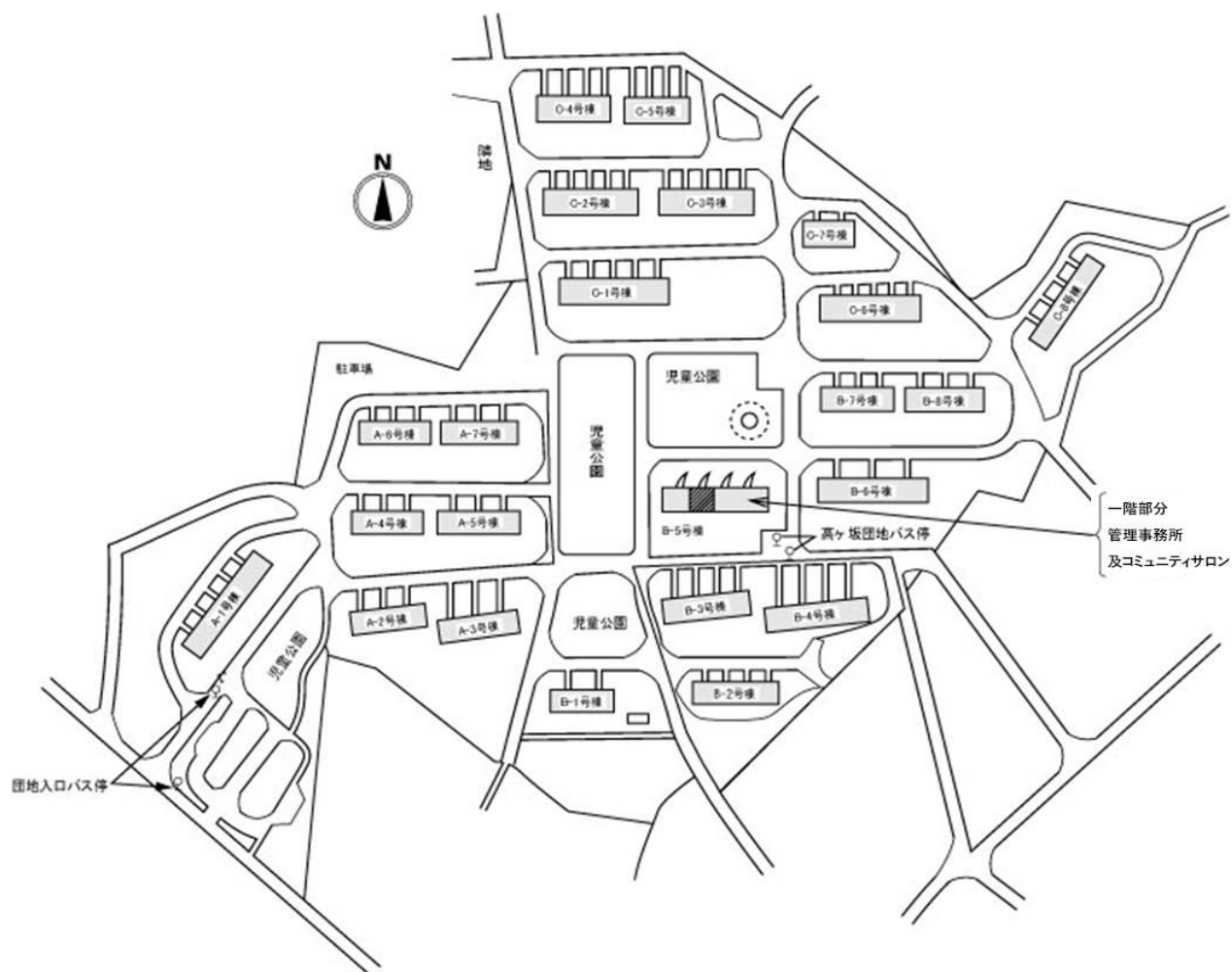
配置図
