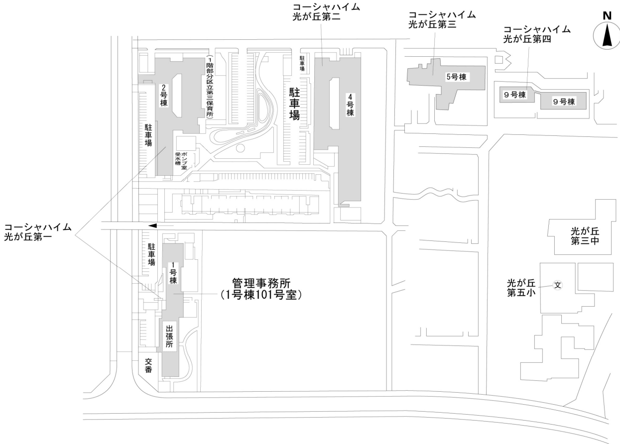
配置図
