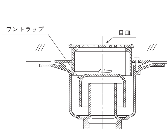
床排水トラップ (椀型)
